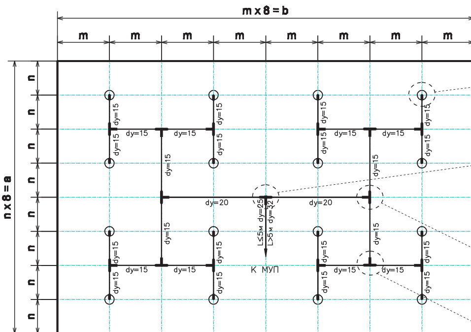
Схема 3 УП ТВ-50 при h < 4,0 \text{ м} S_{\text{защ}} \leq 40 \text{ м}^2
