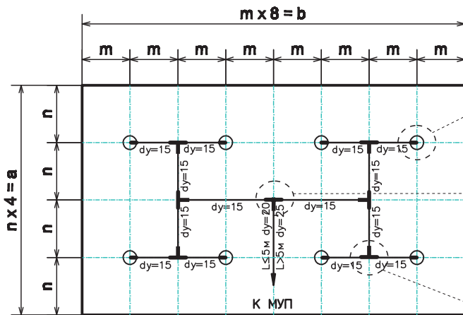
Схема 2 МУП ТВ-27 при 4,0 \text{ м} \leq h < 6,0 \text{ м} S_{\text{защ}} \leq 15 \text{ м}^2
